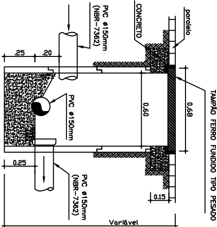
CORTE P.V. ESC.: 1:20
